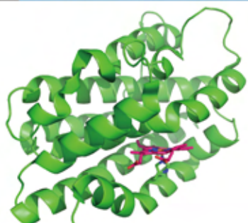
図1 人のヘムオキシゲナーゼの構造
